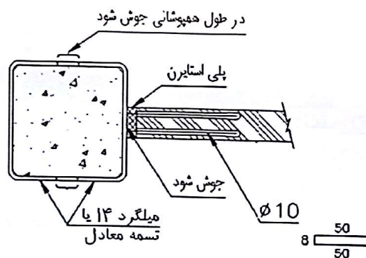
شکل (۴): جزئیات کمربند فلزی و شاخک اتصال
