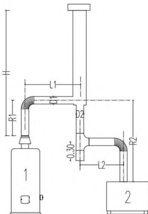
شکل ۱۷-۴-۲ دودکش برای دو یا چند دستگاه گازسوز که در یک طبقه نصب شده‌اند
