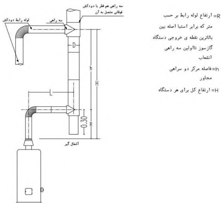
شکل ۳-۴-۱۷ دودکش مشترک در طبقات متوالی ساختمان‌ها
